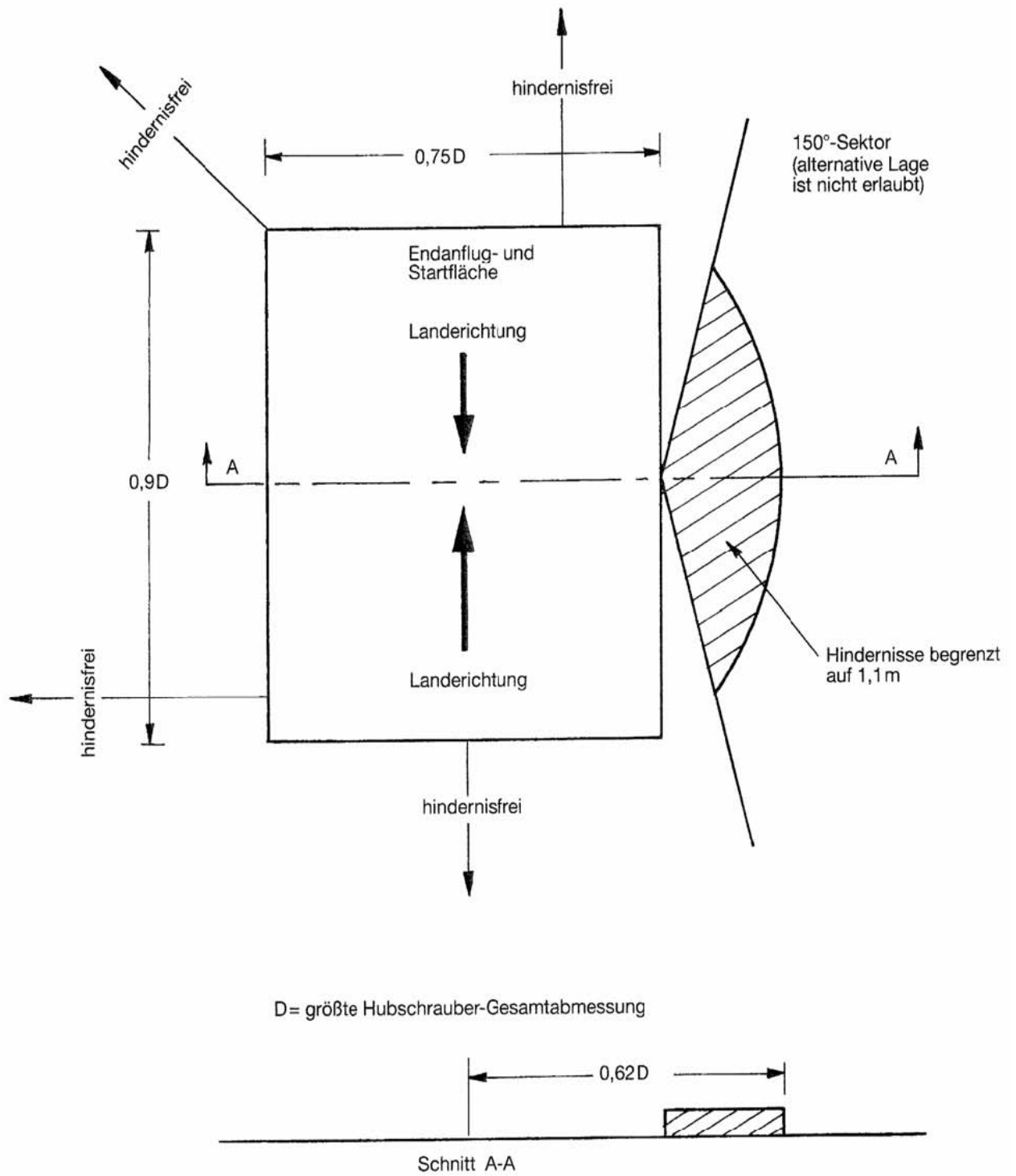
Abbildung 4-5. Hindernisbegrenzungssektoren eines Hubschrauberlandedecks Hubschrauber mit Tandemhauptrotoren – Zweirichtungsbetrieb
