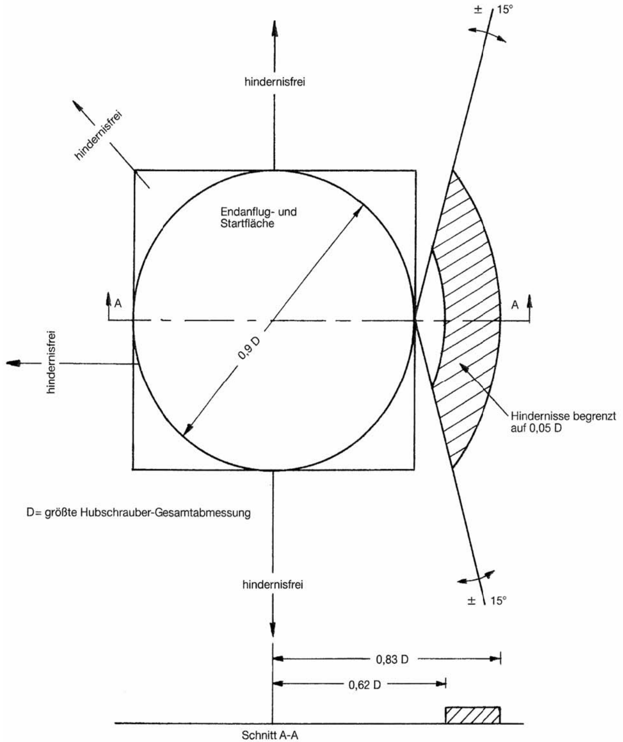
Abbildung 4-4. Hindernisbegrenzungssektoren eines Hubschrauberlandedecks Hubschrauber mit Tandemhauptrotoren – Allrichtungsbetrieb
