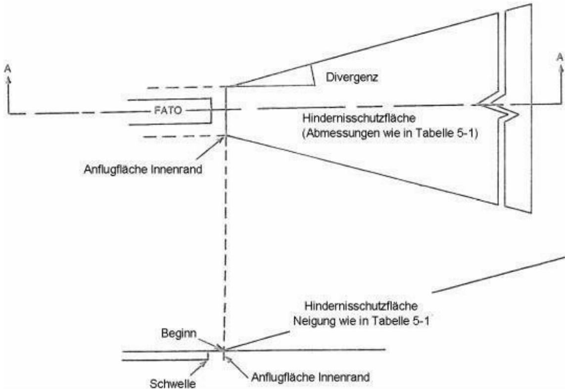
Abbildung 5-12. Hindernisschutzfläche für Gleitwinkelbefeuerungen
